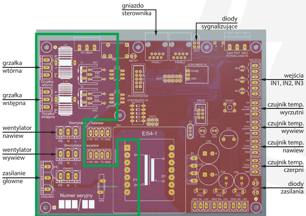
Rys. Schemat sterownika.
