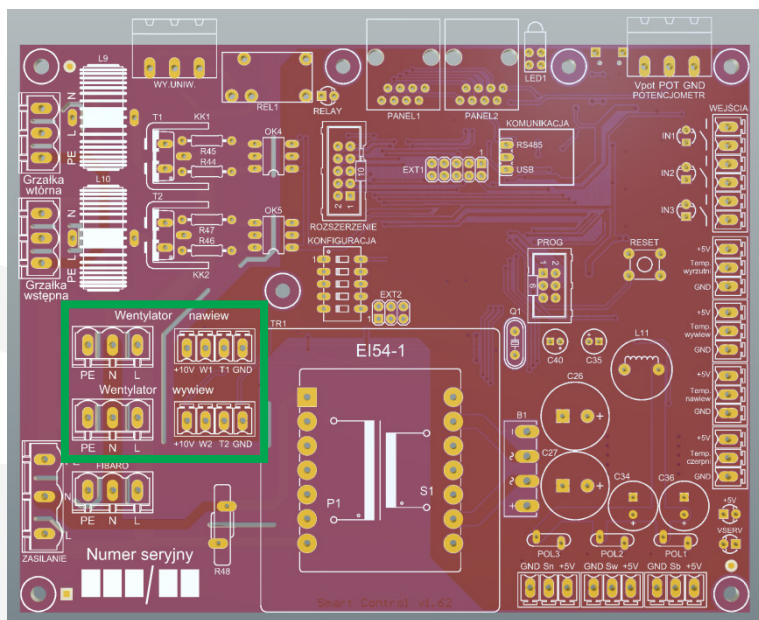
Rys. Schemat podłączenia wentylatorów do sterownika.
