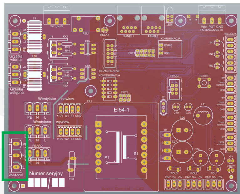
Rys. Schemat podłączenia kabla zasilającego do sterownika.
