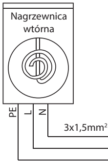
Rys. Schemat podłączenia nagrzewnicy wtórnej.
