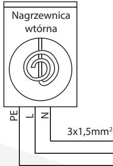
Rys.Schemat podłączenia nagrzewnicy wtórnej.
