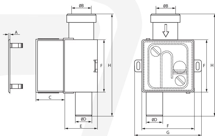
Rys. Syfon kulowy
