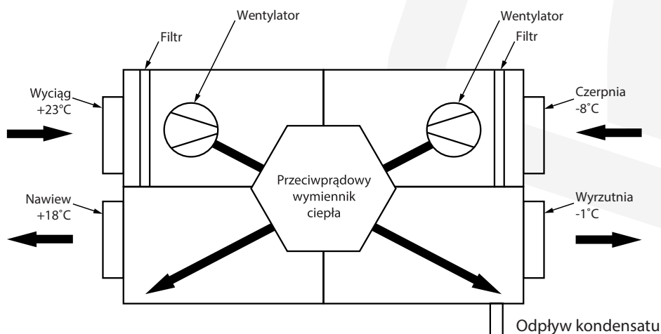
Rys. Zasada działania odzysku ciepła w wymienniku przeciwprądowym
