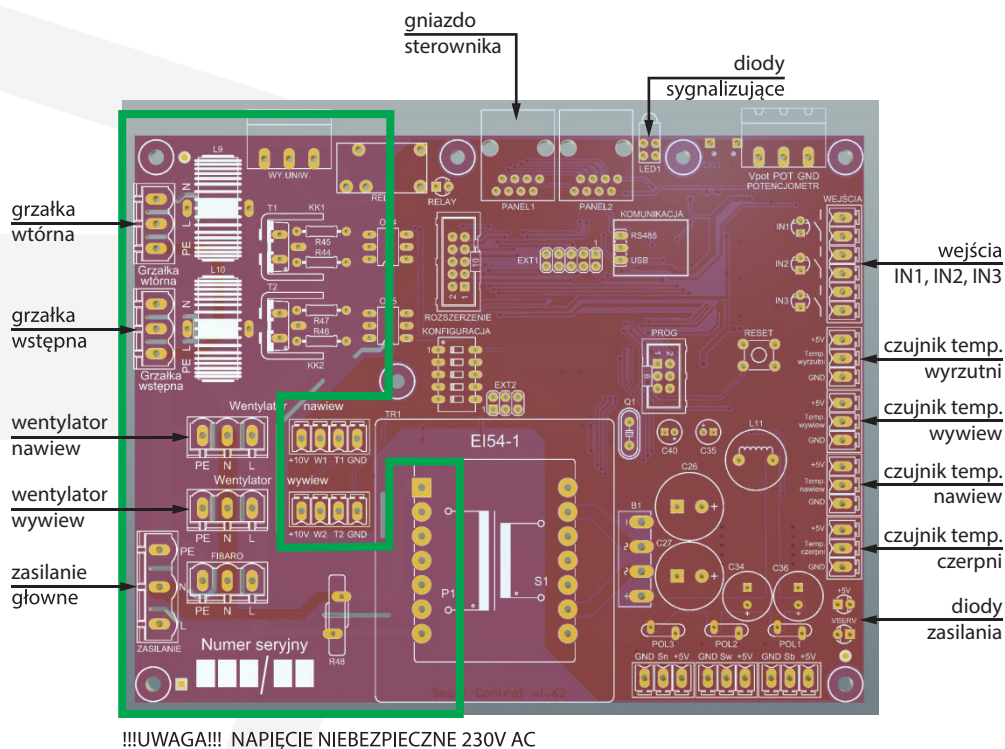
Rys. Schemat sterownika.
